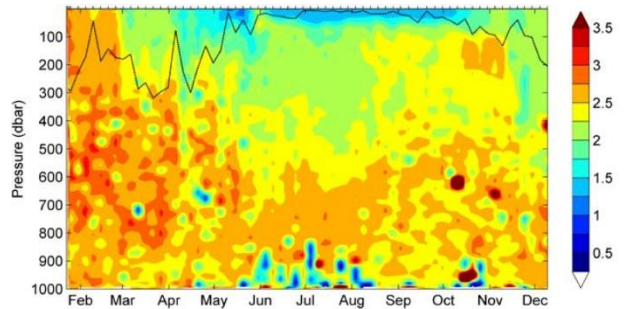
Отношение на коефициента на обратно разсейване при 532 nm и 700 nm ( bbp532/bbp700 ), като функция на дълбочината и времето. Dall'Olmo & Mork (2014)
